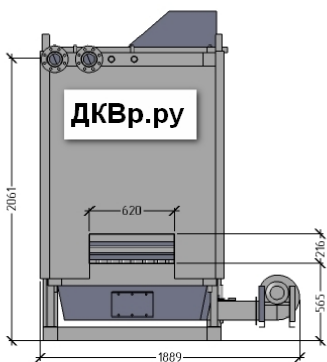
Котел водогрейный КВм-0,35ДВО:
